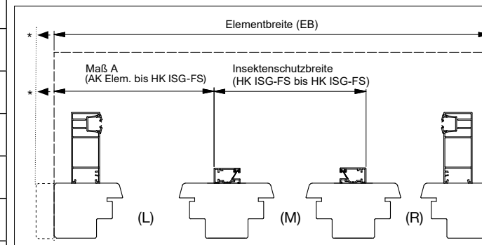
Abbildungen der Führungsschienen beispielhaft, AK Elem. = Außenkante Element * Darstellung bei eingerückter Führungsschiene
