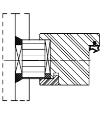
Massivholzstockzarge Schraubbefestigung (Blendrahmenmontage)
