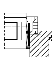
Massivholzstockzarge Schraubankerbefestigung (Leibungsmontage)
