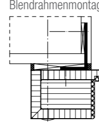
Holzzarge mit angegossener PU-Kante Blendrahmenmontage
