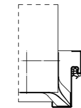
Stahlsanierungseckzarge mit schräger Verschraubung
