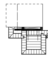
Faltstockzarge Schweißankerbefestigung (Leibungsmontage)
